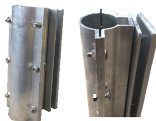
KDE250-Halterung mit 2 Stahlplatten für Befestigung auf Leitschienen
