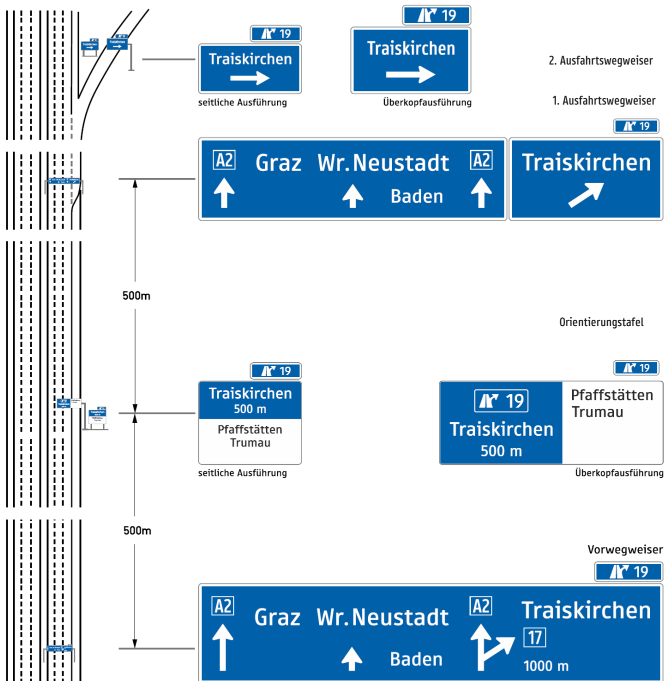
Regelplan Anschlussstelle, RFB mit 3 Fahrstreifen
